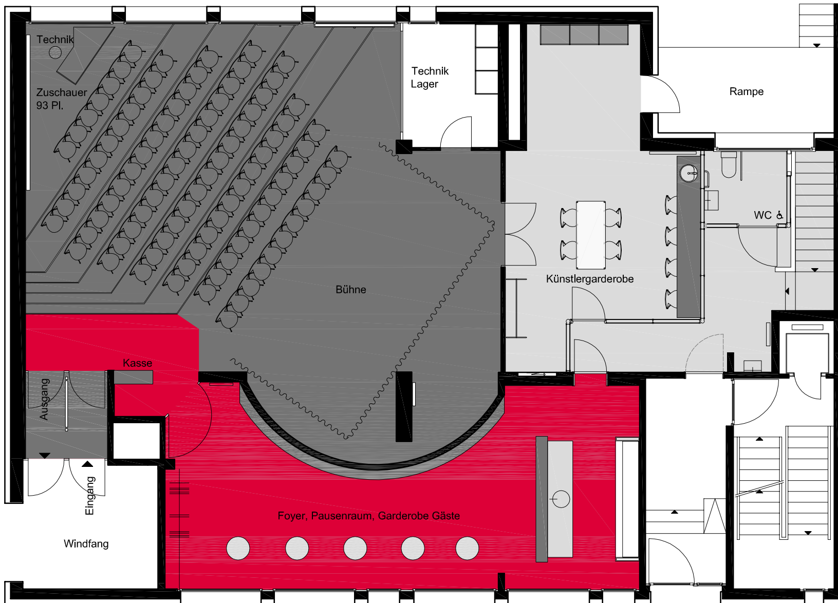
Grundriss Erdgeschoss
