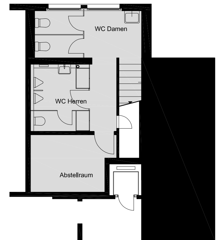
Grundriss Untergeschoss
