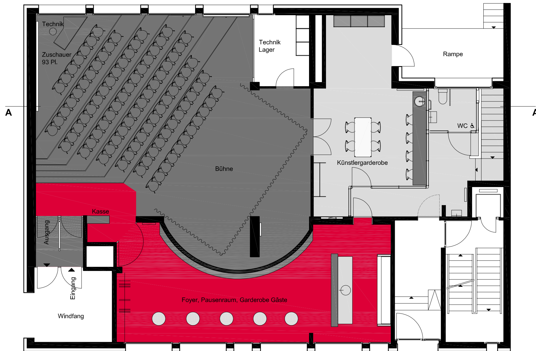
Grundriss Erdgeschoss
